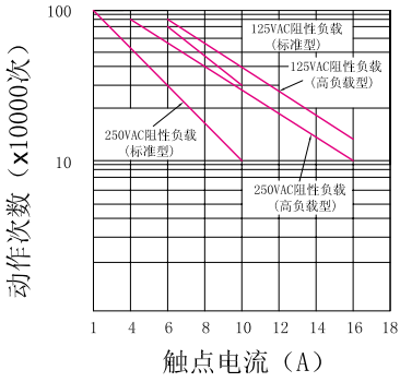
寿命曲线
