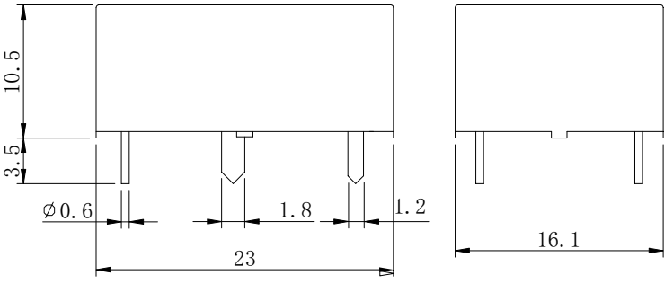
外形图
