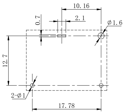
安装孔尺寸图
