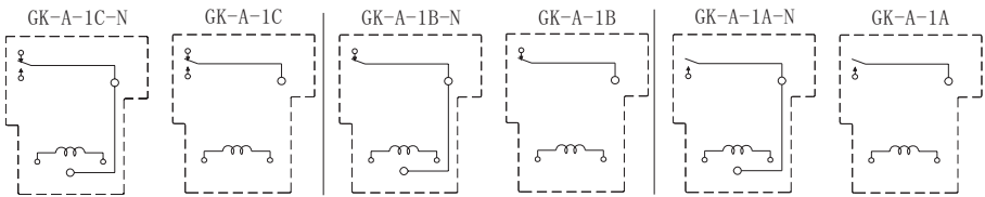
接线图
