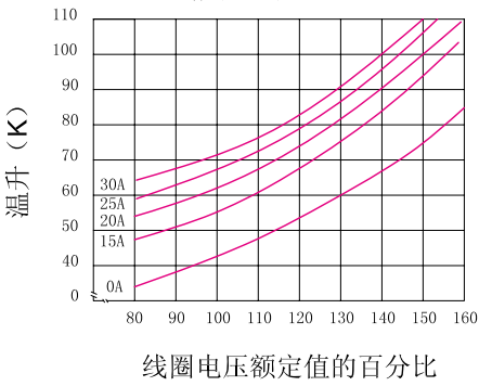
线圈温升
