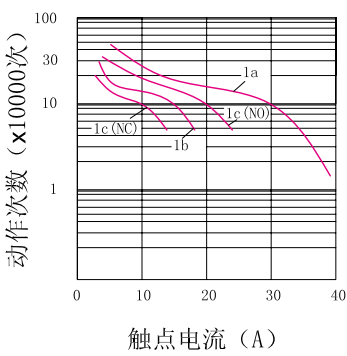
寿命曲线
